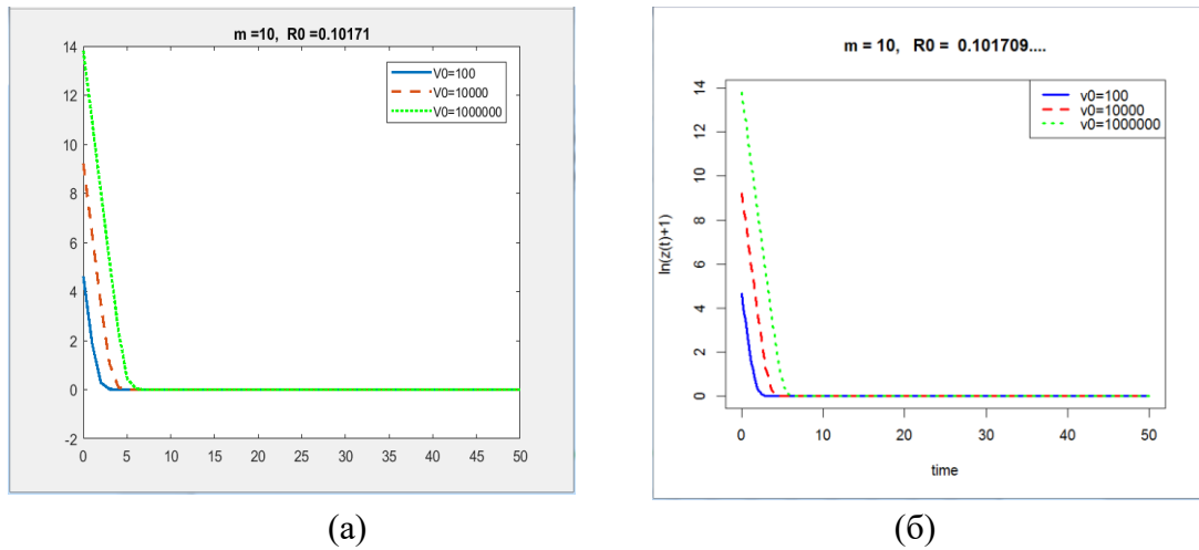
Рис. 1. Динамика \ln(z(t)+1) при V_0 = 10^2, 10^4, 10^6 в MatLab (а) и в пакете R (б) в случае R_0 < 1
